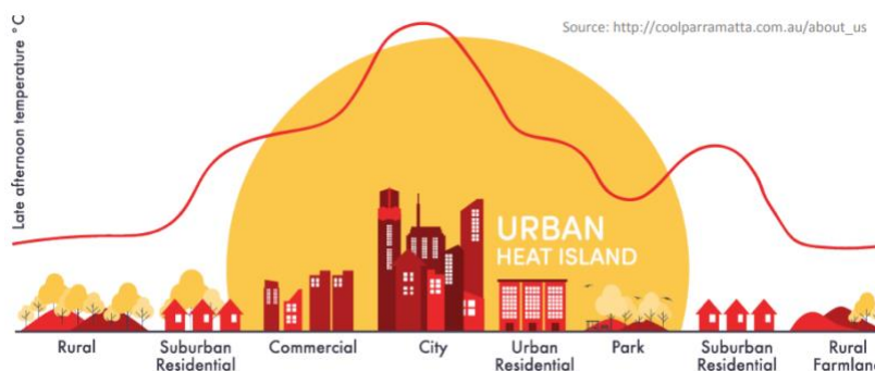
Gambar 1. Ilustrasi Fenomena UHI [7]
