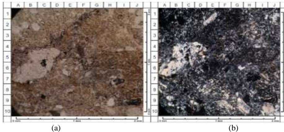
Gambar 2. Kenampakan sayatan tipis batuan di daerah penelitian (a) PPL ( Plane Polarized Light ) dan (b) XPL ( Cross Polarized Light )
