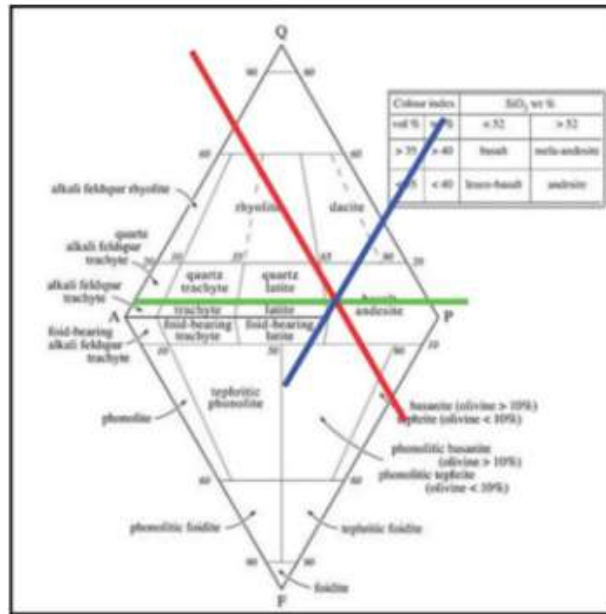
Gambar 3 Ploting hasil analisis petrografis ke dalam klasifikasi Streckeisen (1976)
