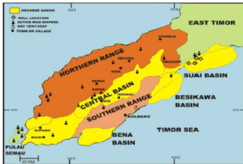
Gambar 2. Peta Zonasi Fisiografi Timor Barat
