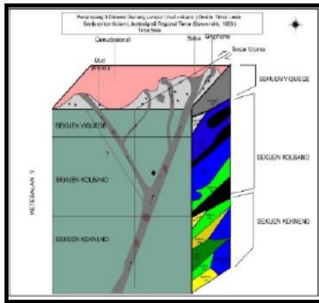
Gambar 5. Model bawah permukaan gunung lumpur
