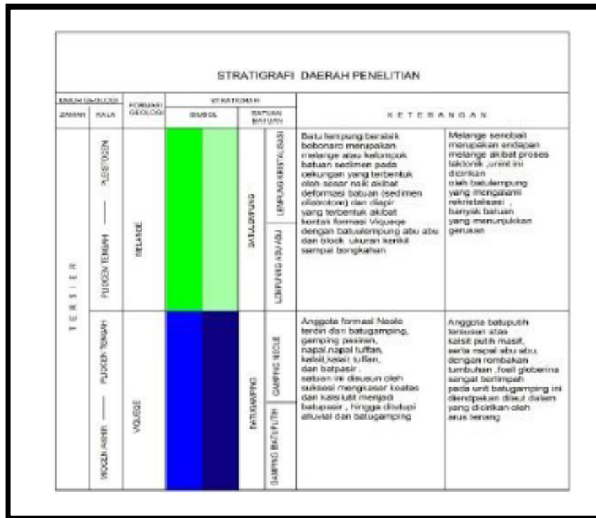
Gambar 4. Stratigrafi daerah penelitian
