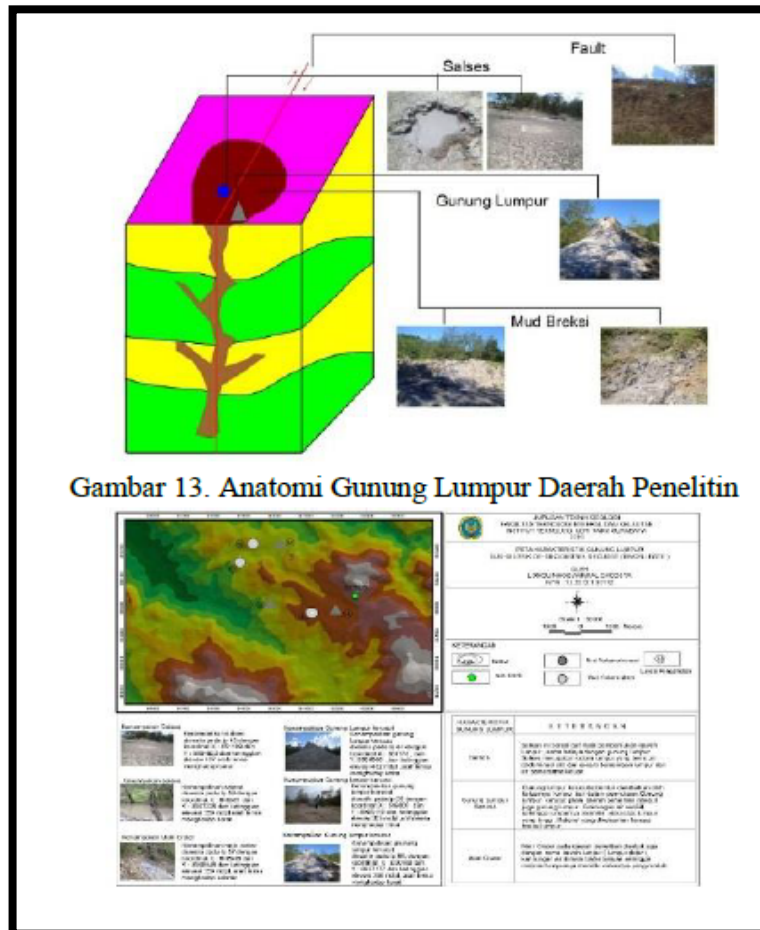
Gambar 10. Anatomi Gunung Lumpur Daerah Penelitian
