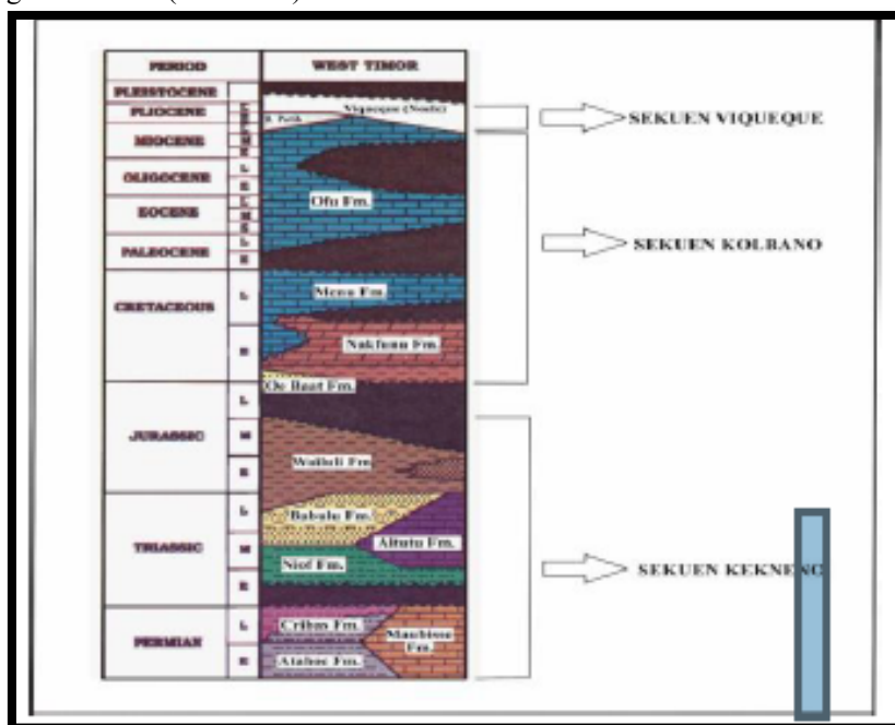
Gambar 3. Kolom litostratigrafi Regional Timor
