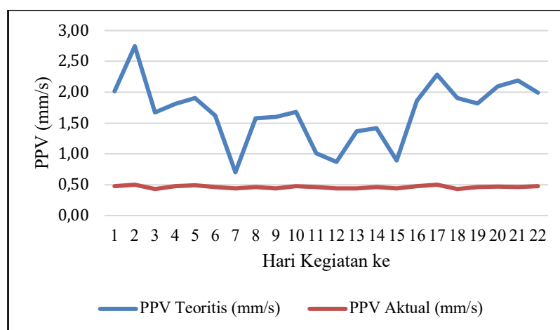
Gambar 5. Grafik Perbandingan antara PPV aktual dan Teoritis
