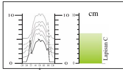
Gambar 8. Kurva distribusi lapisan lanau kasar
