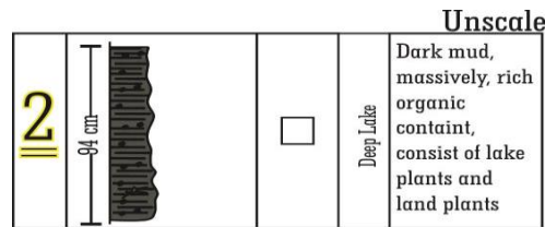
Gambar 11. Kolom stratigrafi dan interpretasi fasies sedimen pada sampel core rwp-02
