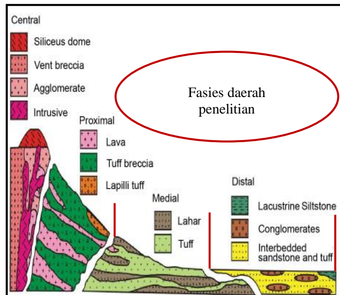
Gambar 5. Pembagian fasies gunungapi pada daerah penelitian [14]
