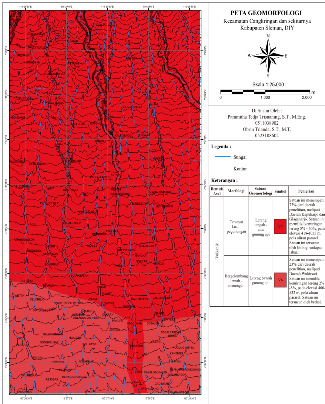
Gambar 2. Pembagian satuan geomorfologi daerah penelitian, lereng tengah atas – bawah (bagian utara; merah tua) dan lereng bawah gunungapi (bagian selatan, merah muda)
